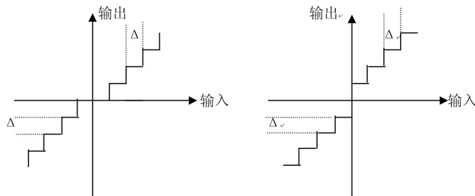
图 5—39 两种均匀量化的输入、输出特性。
