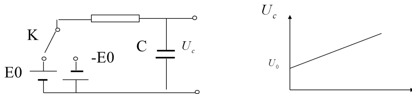
图 5—30 单积分RC译码器
